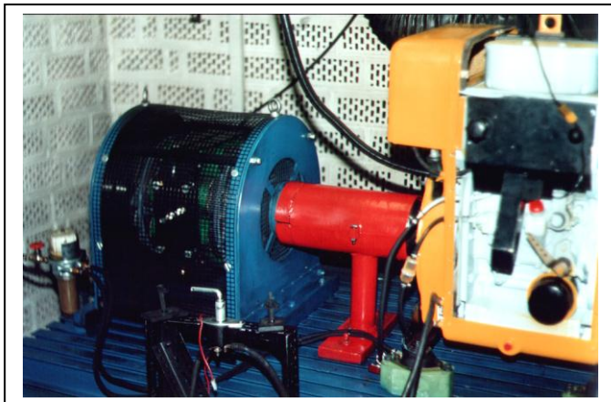
Motorenprüfstand MT 80 für HATZ-Diesel
