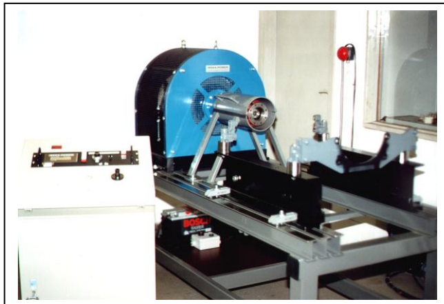
Prüfstand MT 120 für 4 Zyl. DEUTZ-Diesel
